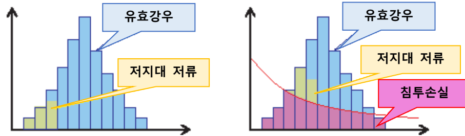
유효강우의 개념
