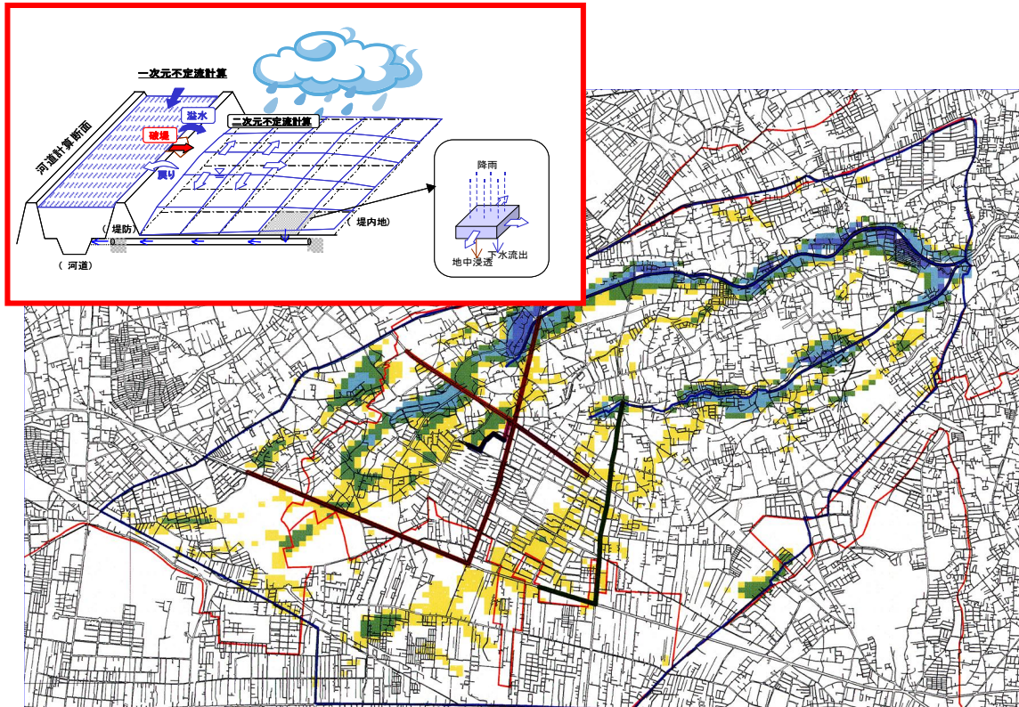
배수시설을 고려한 범람해석 사례
