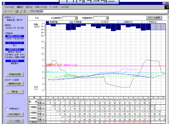
수위예측그래프
