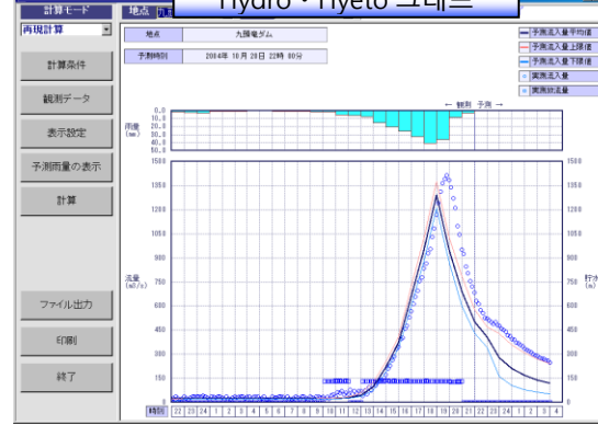
Hydro · Hyeto 그래프
