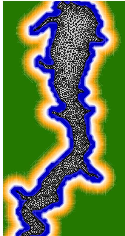
저수지의 격자작성 예(비구조격자)
