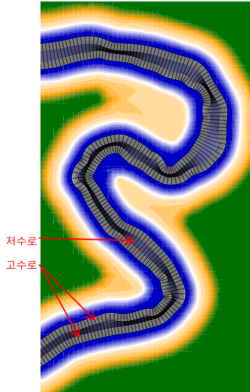
하도의 격자작성 예(직교곡선)
